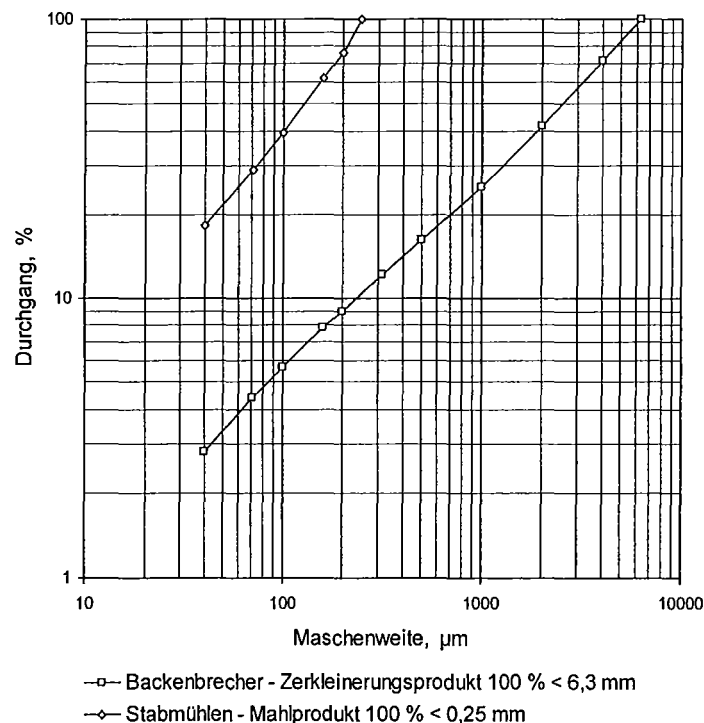
Abb. 1: Siebanalyse des Backenbrecher-Zerkleinerungsproduktes 100% <6,3 mm und des Stabmühlenmahlproduktes 100% <250 µm.
